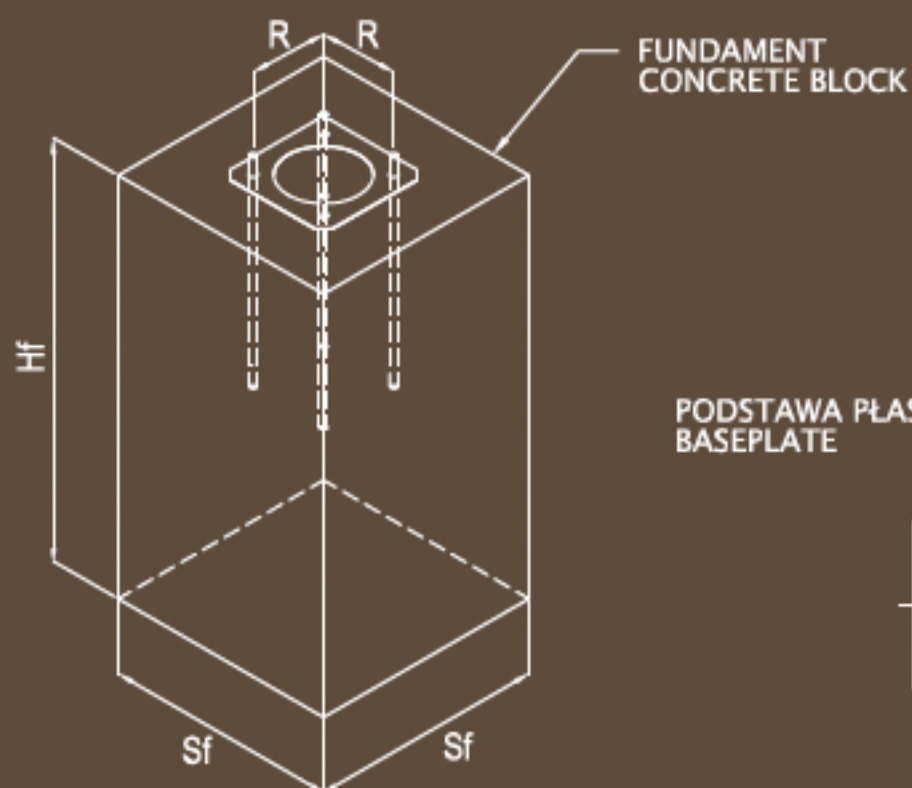
SZCZEGÓŁ POŁĄCZENIA CONNECTION DETAILS
