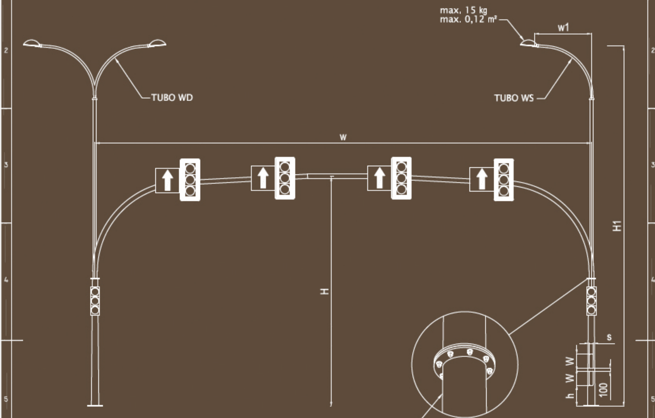
SZCZEGÓŁ POŁĄCZENIA CONNECTION DETAILS
