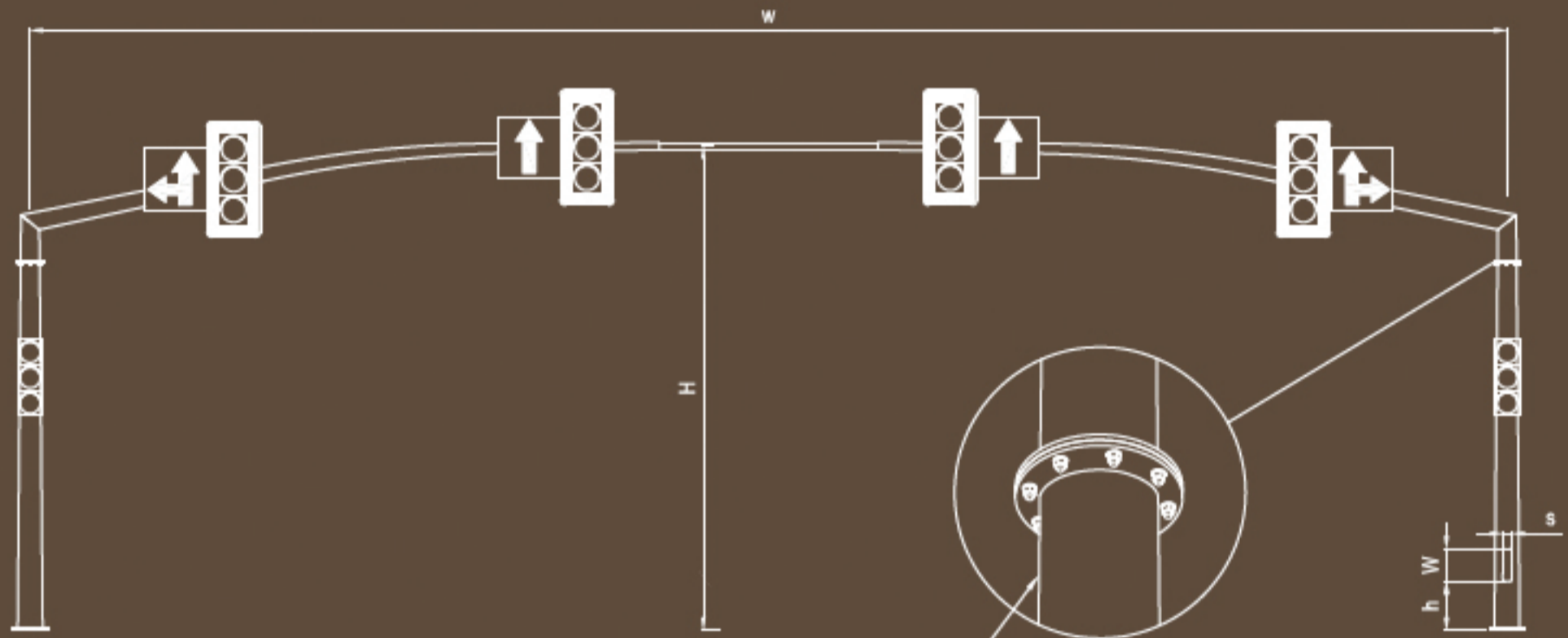
SZCZEGÓŁ POŁĄCZENIA CONNECTION DETAILS
