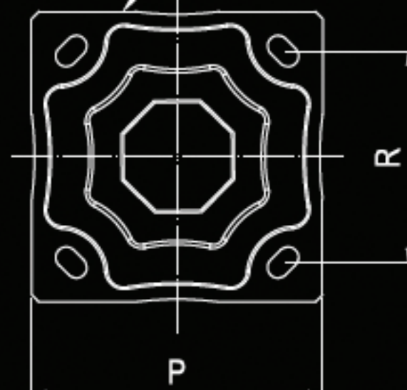
PODSTAWA PRZETŁACZANA STAMPED BASEPLATE
