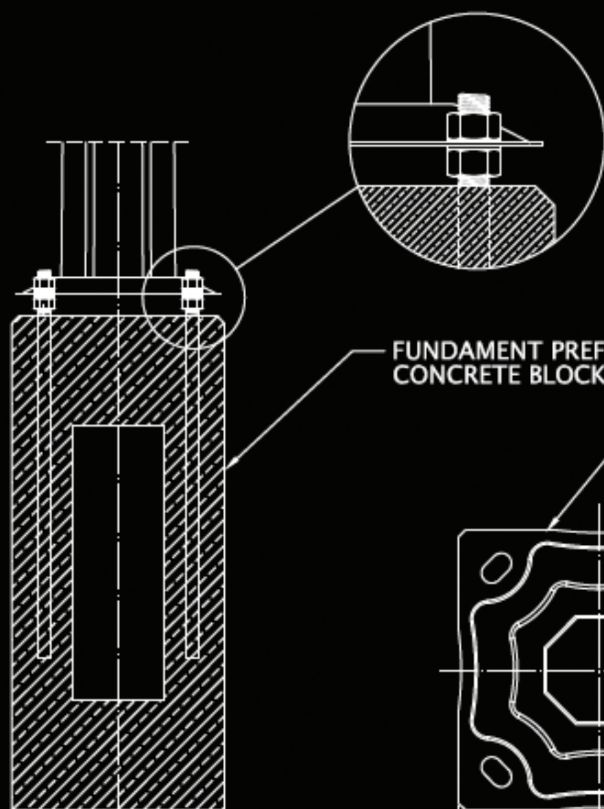
PODSTAWA PRZETŁACZANA STAMPED BASEPLATE
