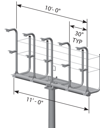
T15 CAGE (15 Luminaires)
