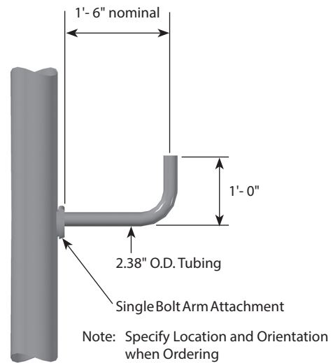
M080 ARM
