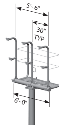
W9 CAGE (9 Luminaires)
