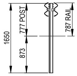
SECTION D-D SCALE 1 : 50
