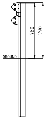
SECTION A-A 1:20
