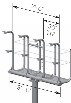
B12 CAGE (12 Luminaires)
