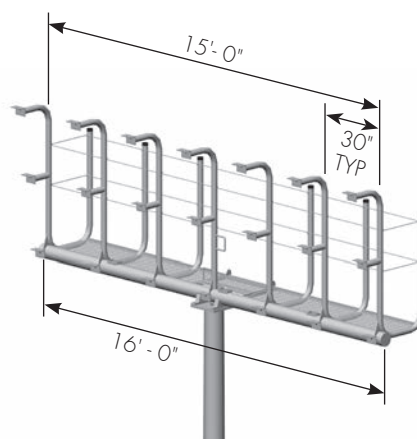
Y21 CAGE (21 Luminaires)
